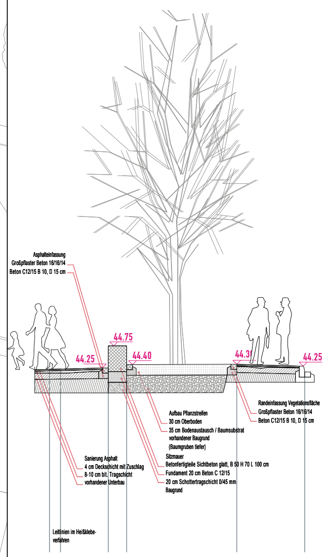
Schnitt A-A Hochbeet, Einfassungen M 1:10
